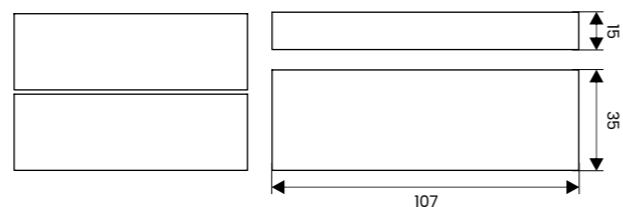
Wymiary oraz schemat ułożenia elementów na palecie.
