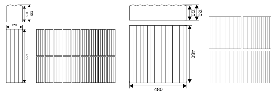
Matmenys ir elementų išdėstymo ant padėklo schema. Dėmesio. Atskiri elementai nėra parduodami vienetais.
