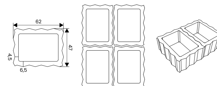
Matmenys ir elementų išdėstymo ant padėklo schema. Dėmesio. Atskiri elementai nėra parduodami vienetais.
